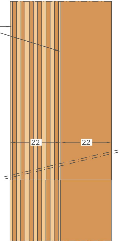
SEZIONE VERTICALE Vertical cross section
